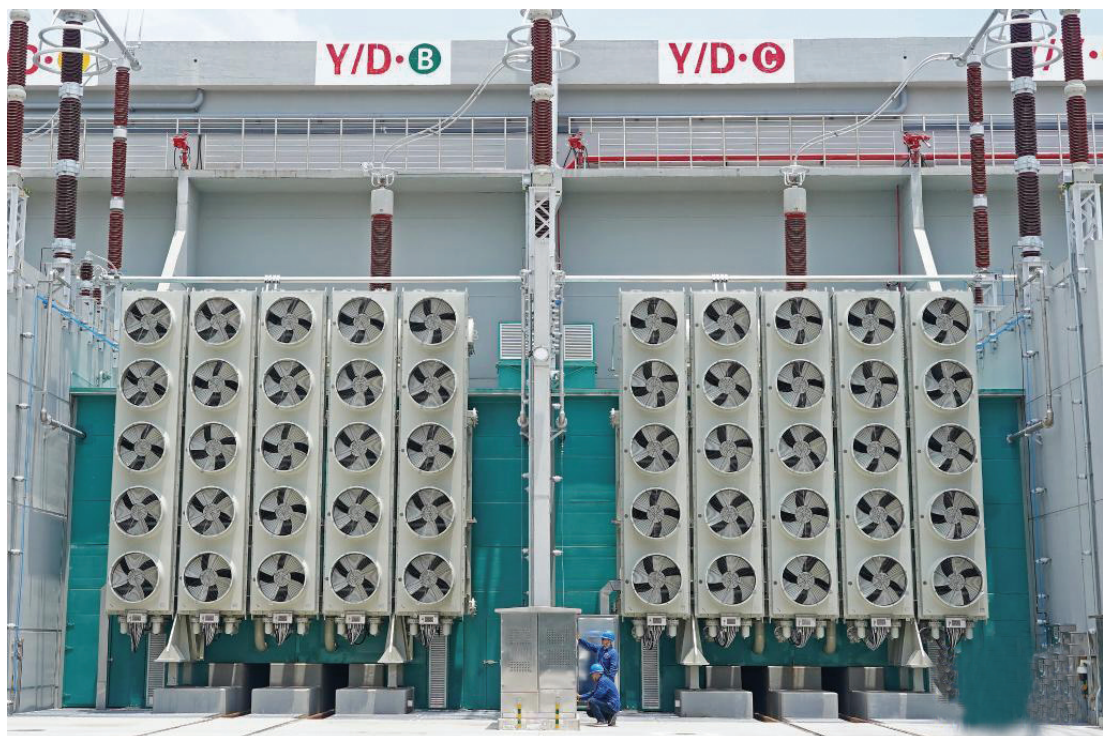
6月21日,四川雅中到江西都阳湖±800千伏特高压直流输电工程正式投运。该工程是国家电网“西电东送”能源战略的重大项目,途经四川、云南、贵州、湖南、江西5省,全线总长约1696千米,设计年输送电量360亿千瓦时。图为工作人员在换流站检查换流变运行状态。新华社记者 万象 摄
