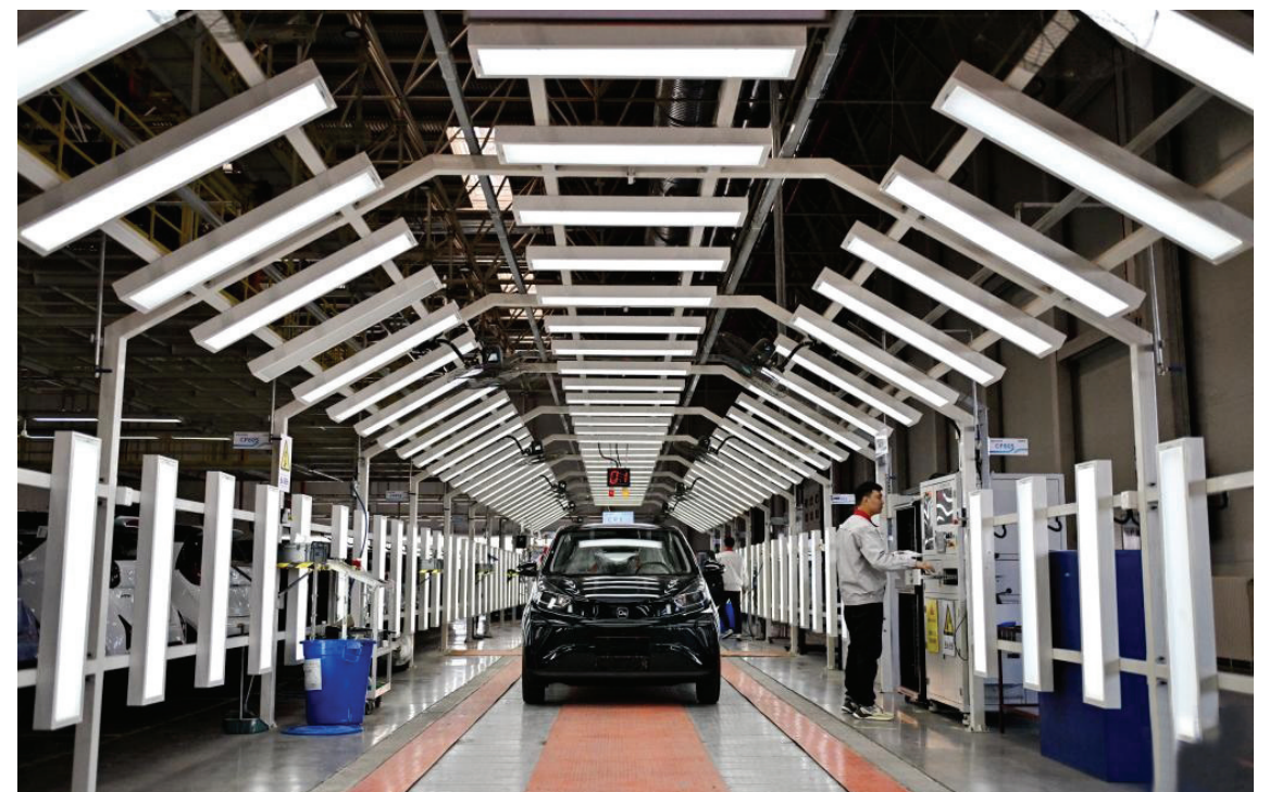
3月19日,奇瑞新能源汽车股份有限公司石家庄分公司的工人在总装车间检测线上工作。
